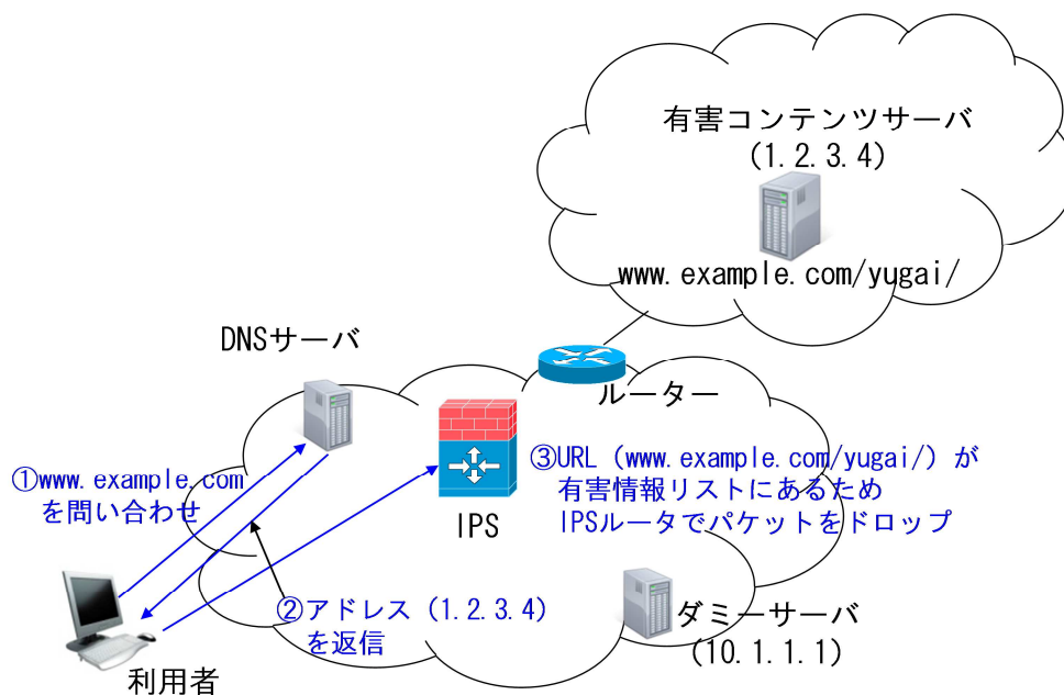
図4 URL フィルタリング
