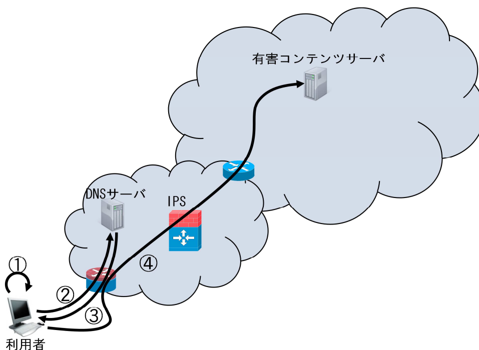
図1 インターネットでの通信の仕組み
