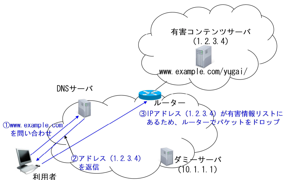
図3 パケットドロップ方式
